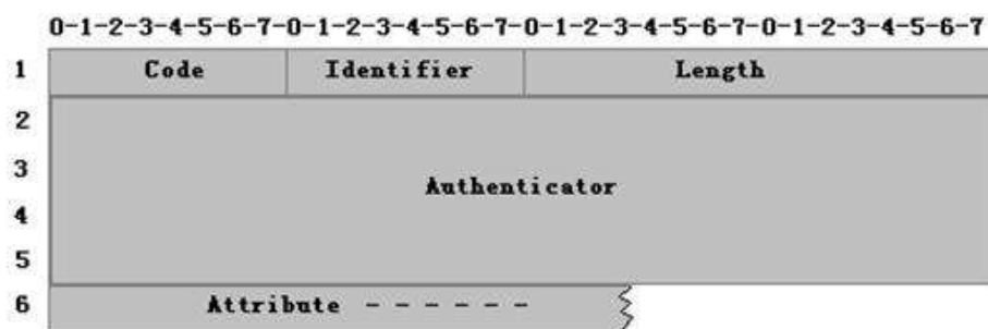
RADIUSMessage format
